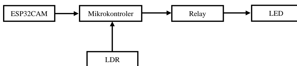
Gambar 2. Diagram Blok Alat (Sumber : dokumen pribadi)
