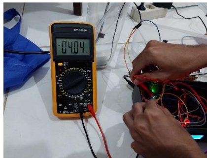
Gambar 10. Pengukuran Tegangan Pada Komponen Relay Yang Terhubung Dengan Pompa Air
